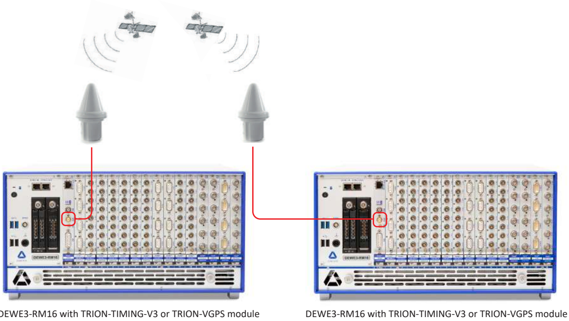
Fig. 22: GPS sync
