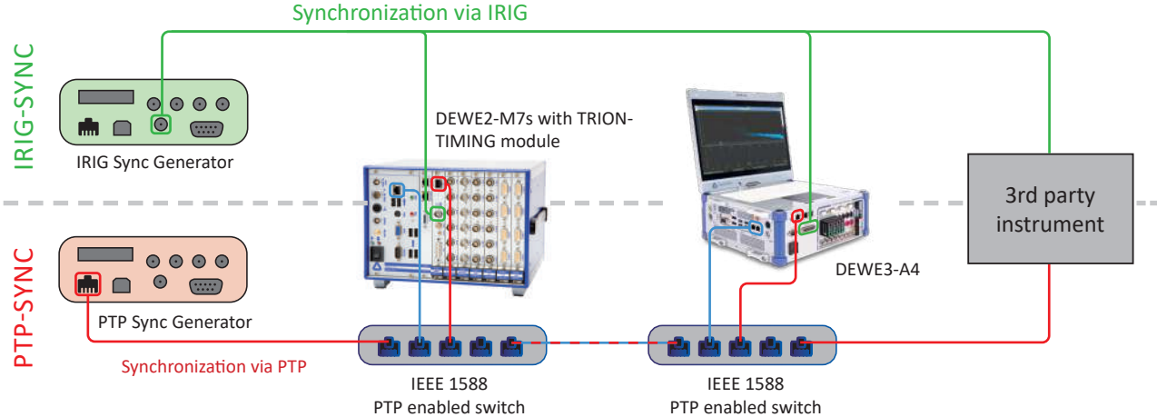
Fig. 25: PTP sync / IRIG sync
